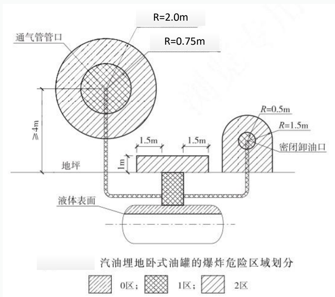
图3 埋地卧式车用乙醇汽油储罐爆炸危险区域划分
