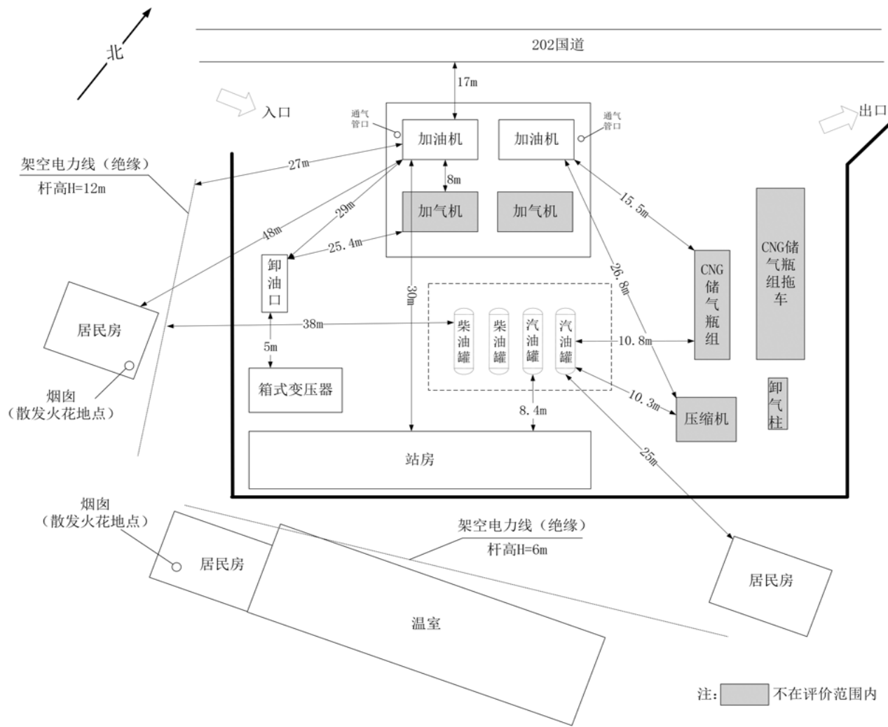
图 2.3-1 清原加油站周边环境和总平面布置示意图
