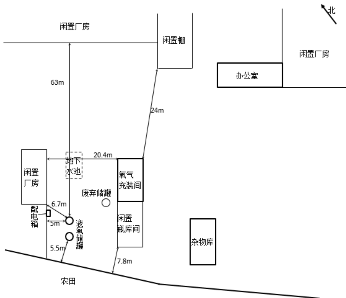
图 2.2-2 企业周边环境示意图
