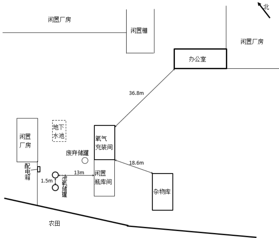
图 2.3-1 总平面布置简图
