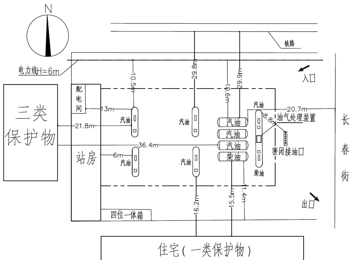
图 2.3-1 周边环境和总平面布置示意图
