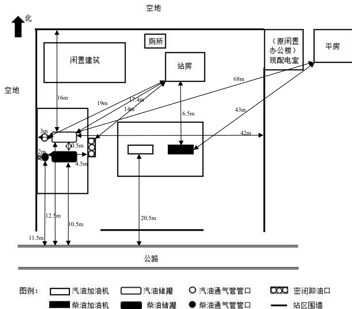
图 2.3-1 周边环境及总平面布置图
