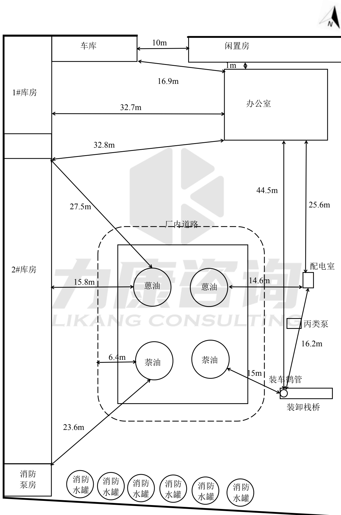
图 2.3-4 企业平面布置图
