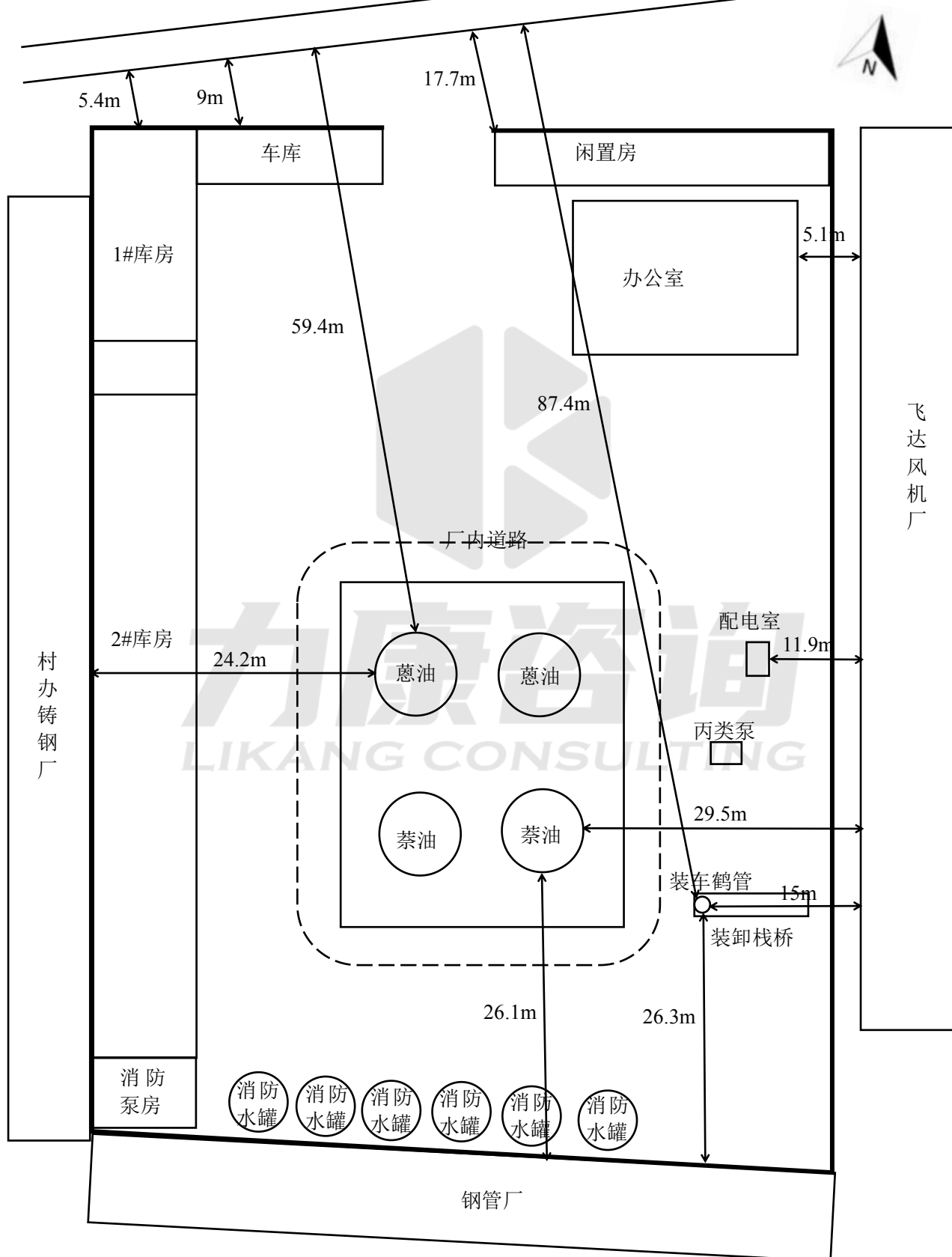
图 2.3-3 企业周边环境示意图
