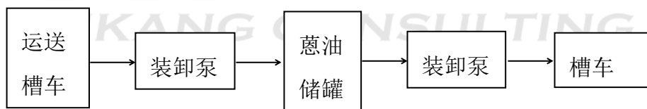
图 2.3-5 葱油装卸流程示意图
