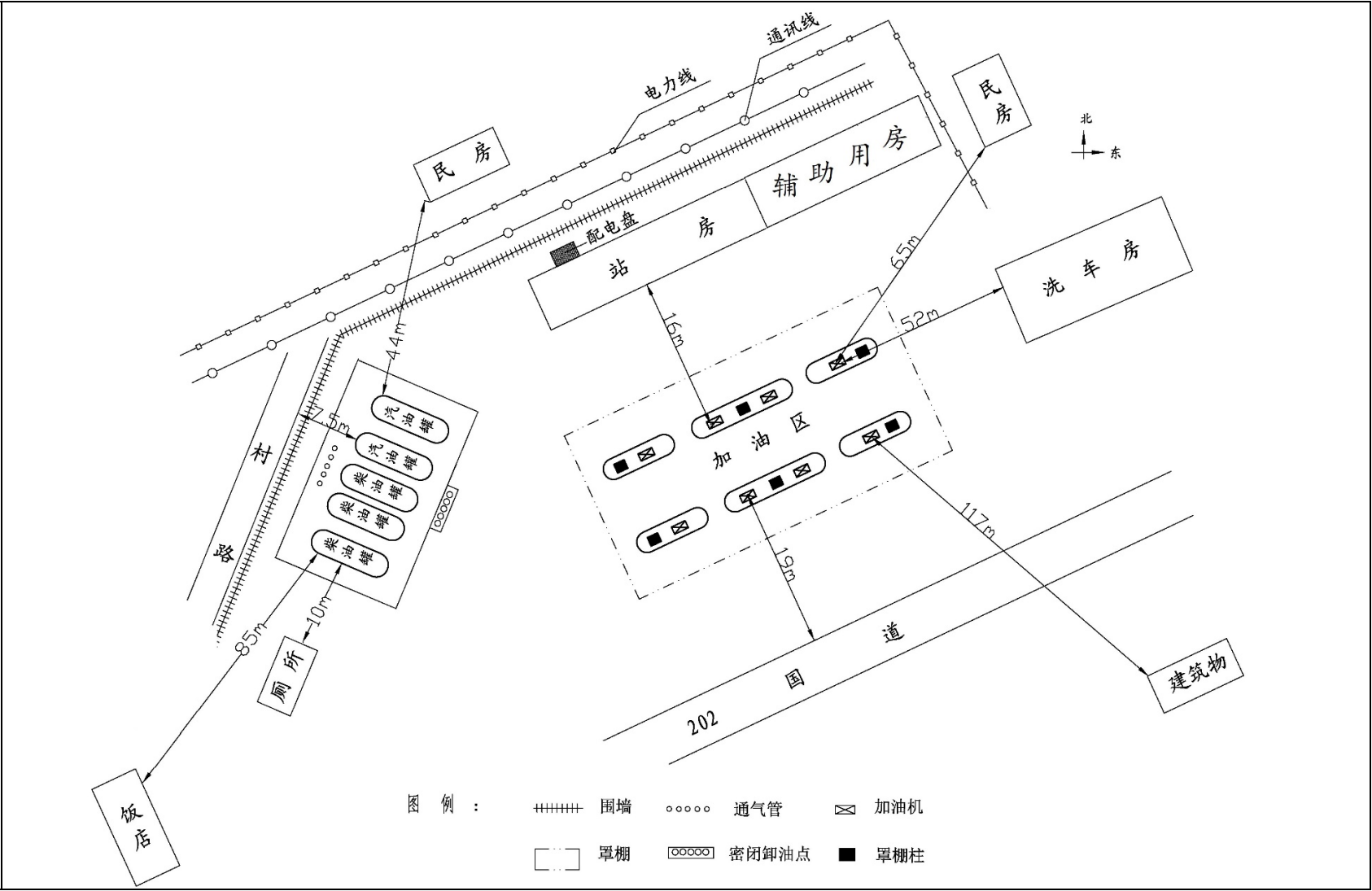
图 2.3-1 周边环境及总平面布置图
