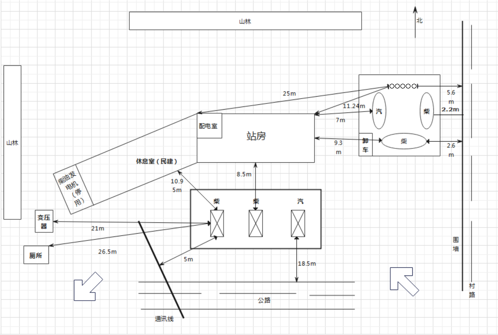
图 2.3-1 周边环境和总平面布置示意图
