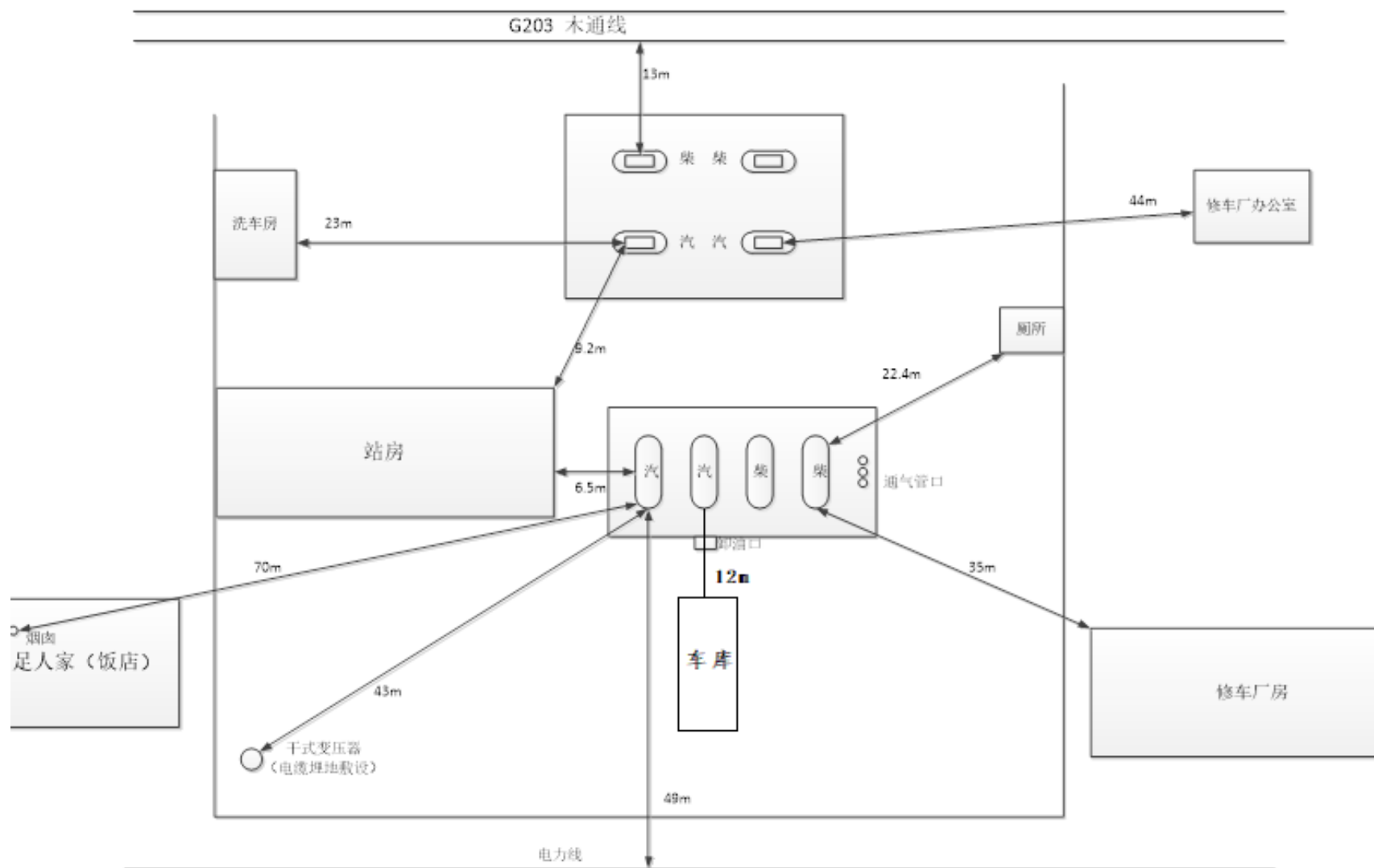
图 2.3-1 周边环境和总平面布置示意图
