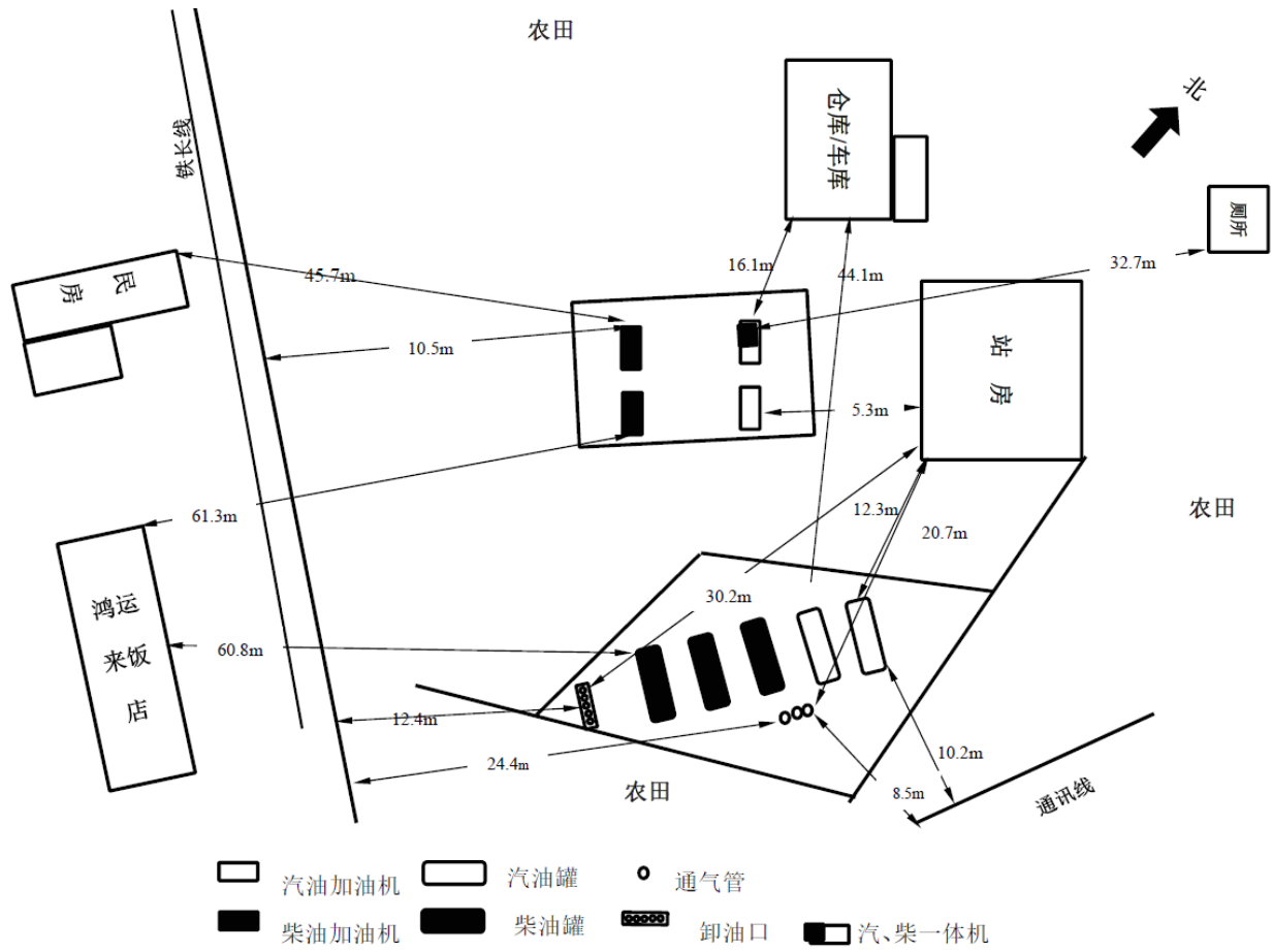
图 2.3-1 周边环境和总平面布置示意图
