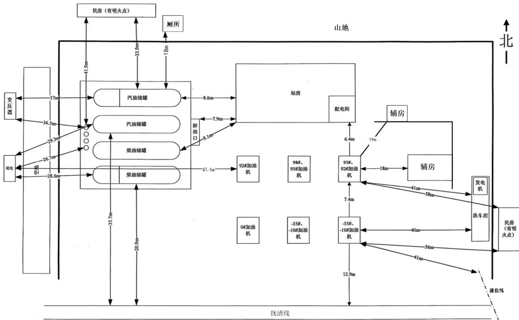
图 2.3-1 加油站周边环境和总平面布置示意图
