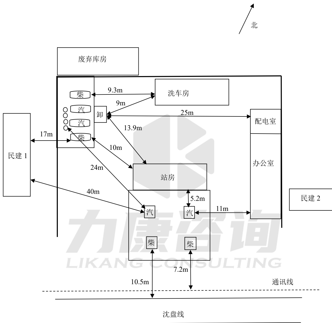
图 2.3-1 周边环境及总平面示意图
