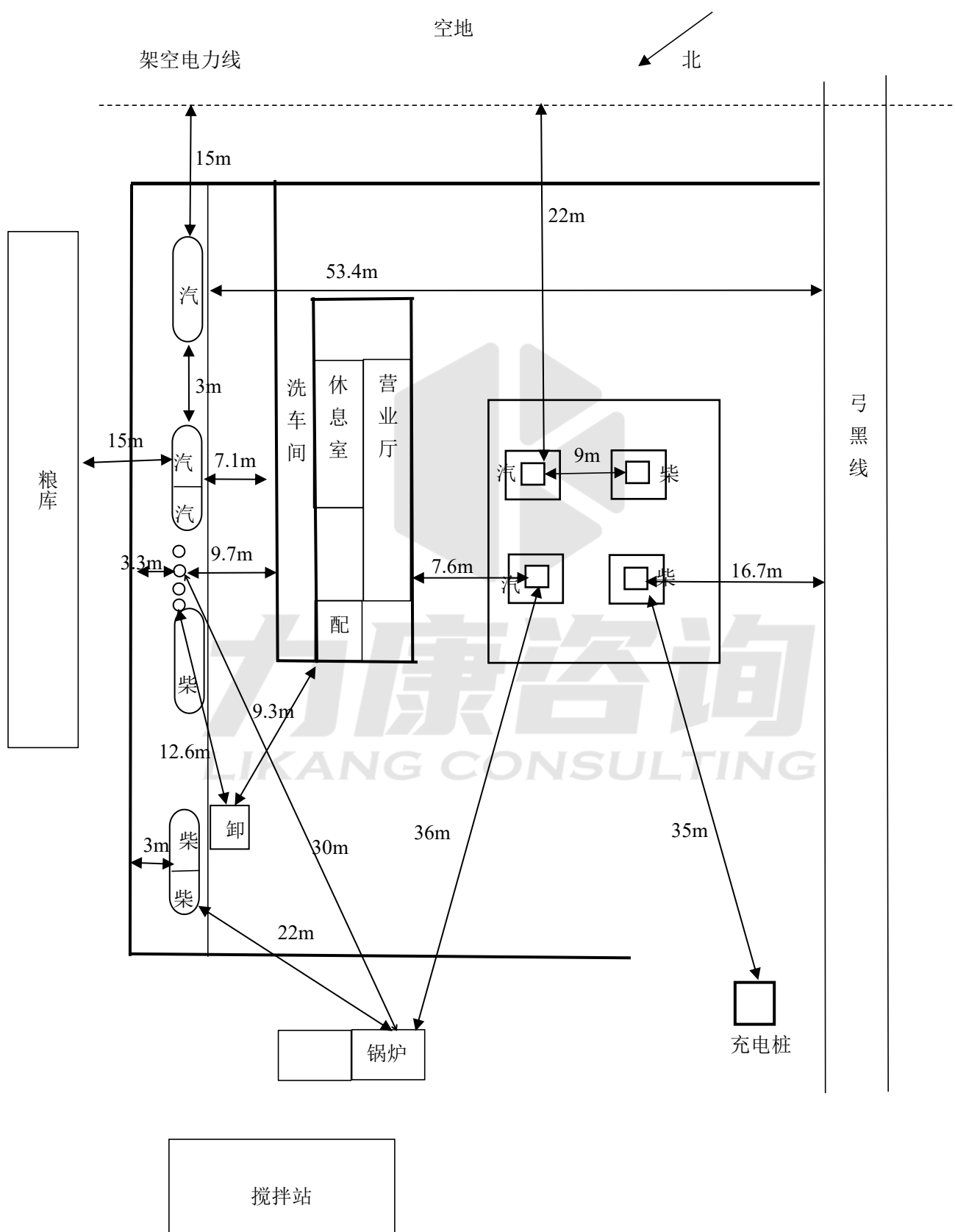
图 2.3-1 周边环境及总平面示意图
