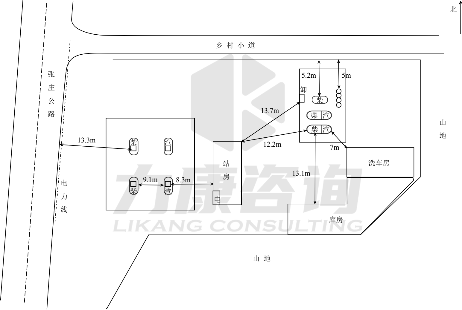
图 2.3-1 周边环境及总平面示意图
