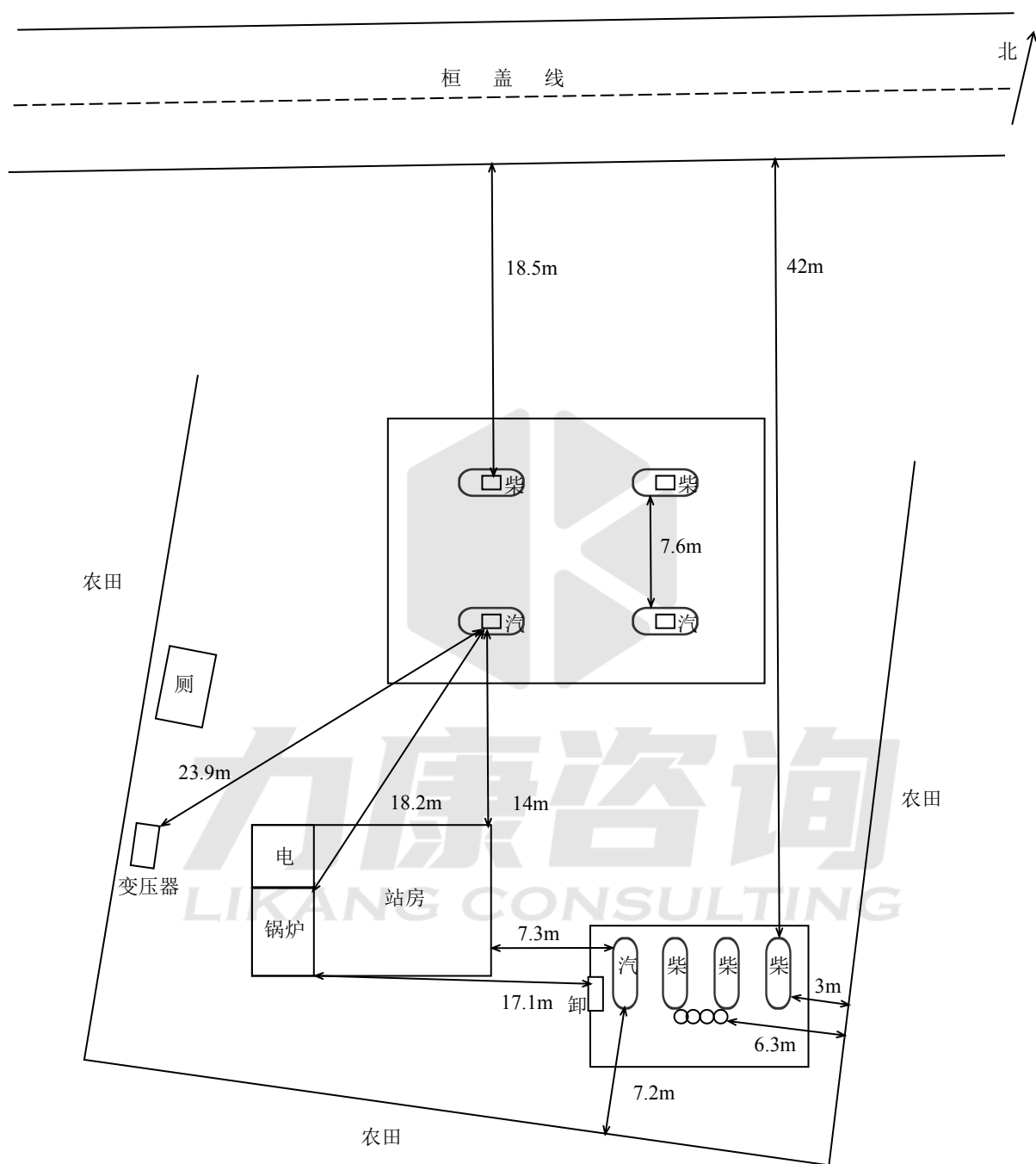
图 2.3-1 周边环境及总平面示意图
