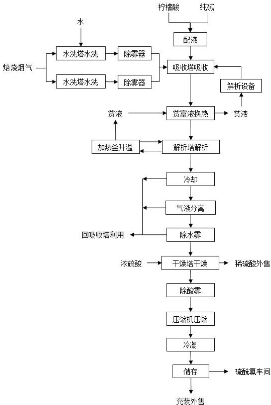
图 2.5-1 改扩建前二氧化硫回收工艺流程示意图
