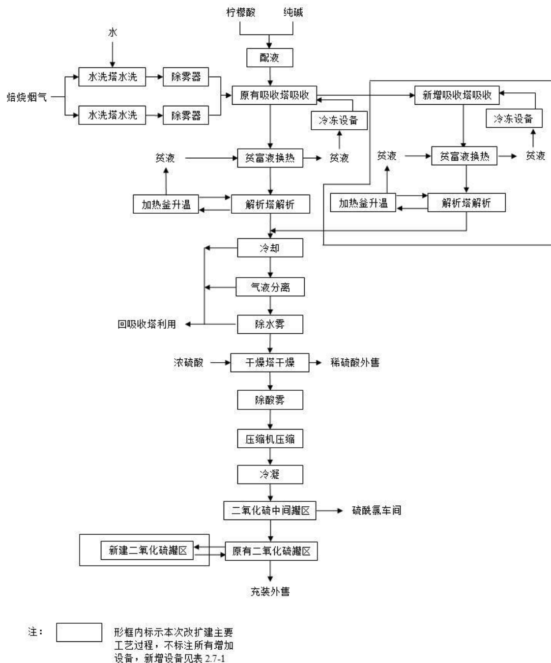
图 2.5-2 改扩建后二氧化硫回收工艺流程示意图
