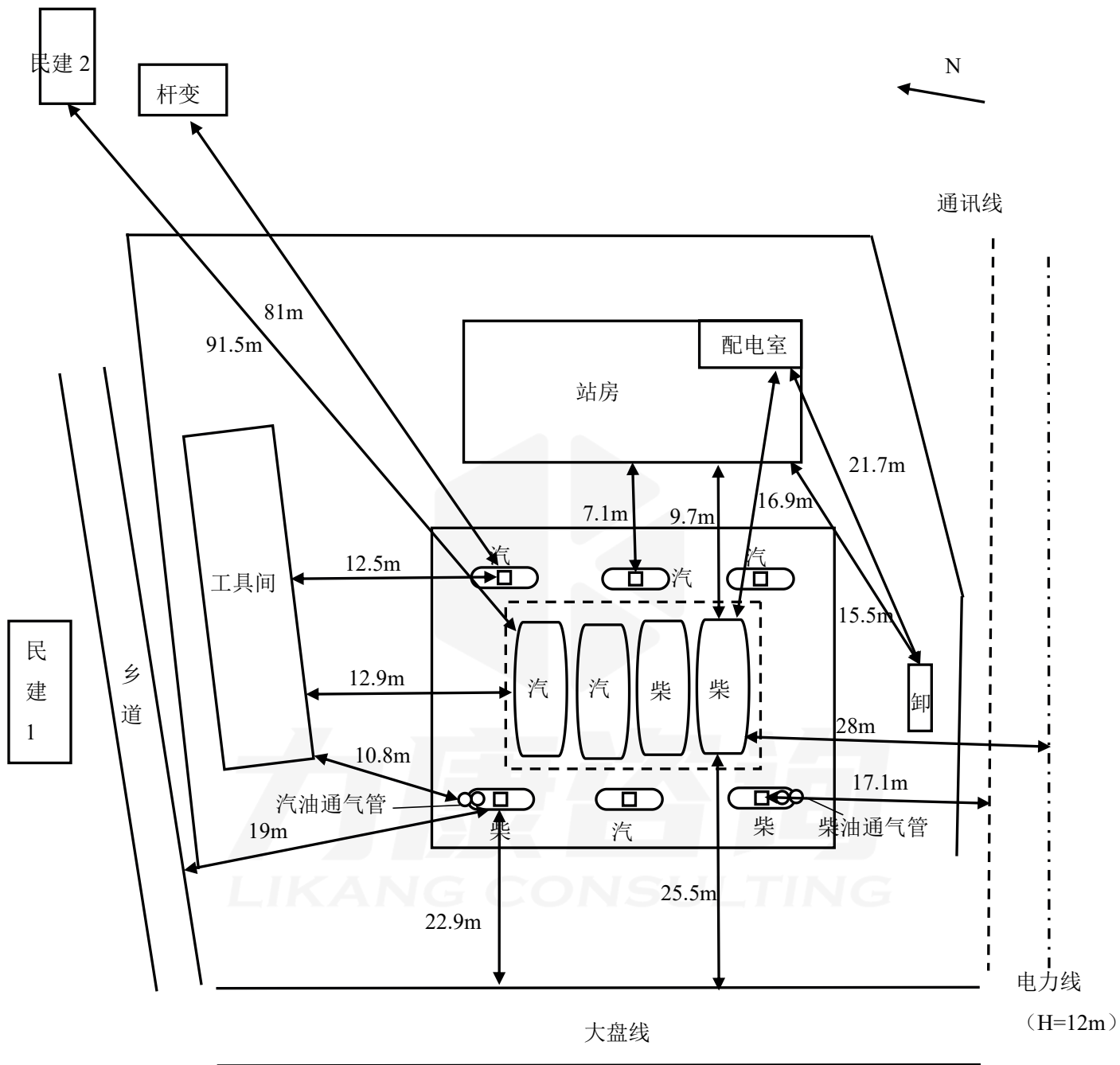
图 2-7 加油站平面布置示意图
