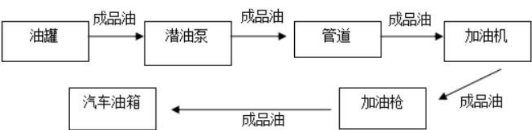
图 2-6 柴油加油工艺过程图
