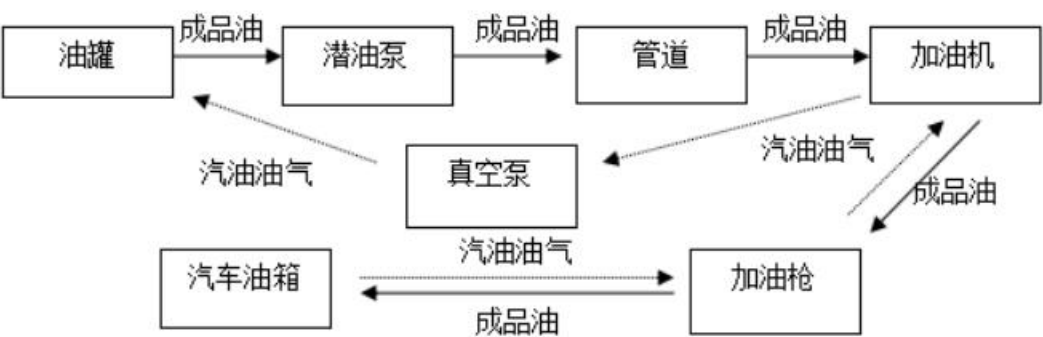
图 2-5 汽油加油及加油油气回收工艺流程
