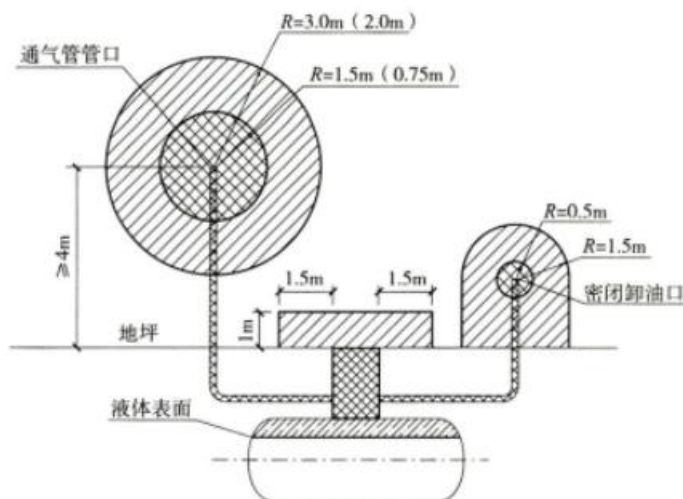
图 5-3 埋地卧式车用乙醇汽油储罐爆炸危险区域划分
