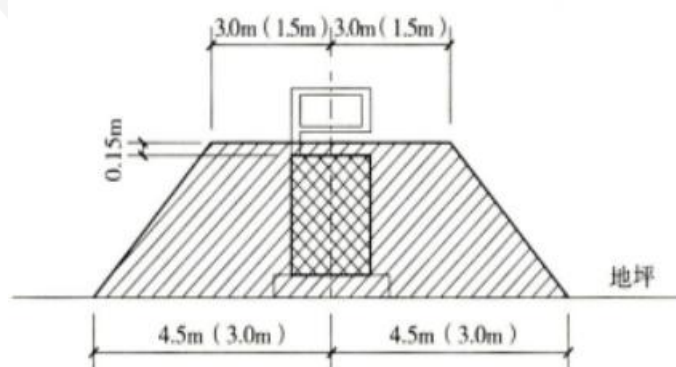
图 5-1 车用乙醇汽油加油机爆炸危险区域划分
