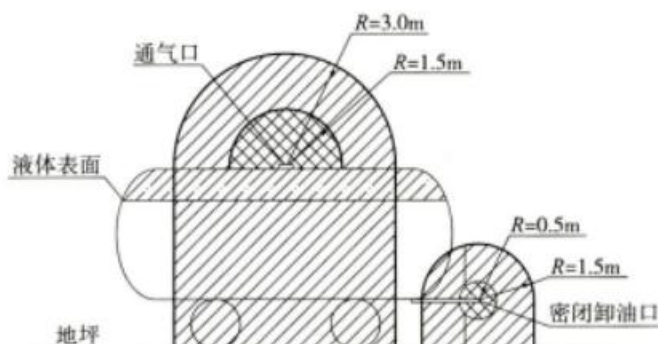
图 5-2 油罐车卸车用乙醇汽油时爆炸危险区域划分
