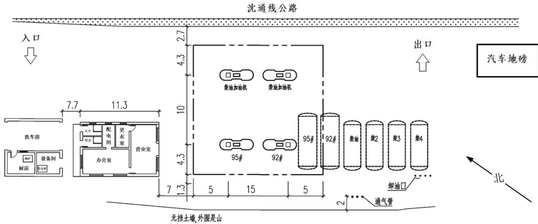
图 2.3-1 加油站周边环境和总平面布置示意图
