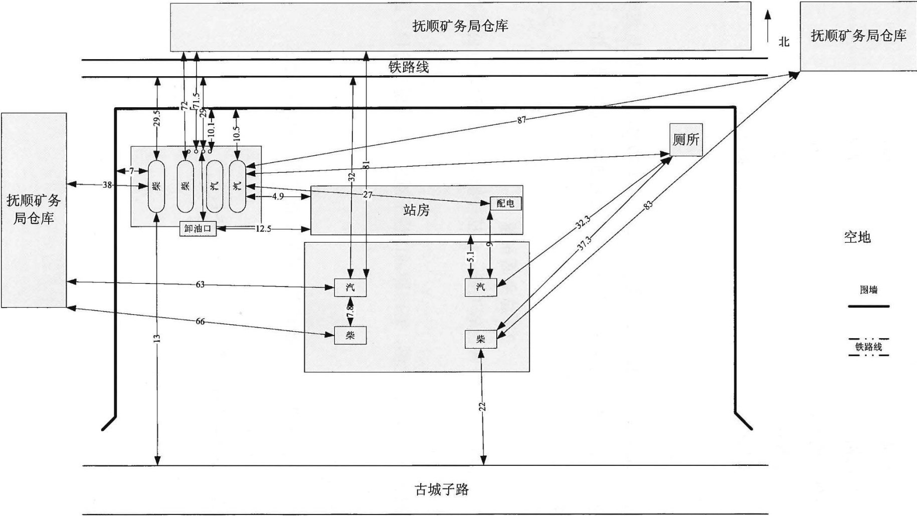
图 2.3-1 加油站周边环境和总平面布置示意图
