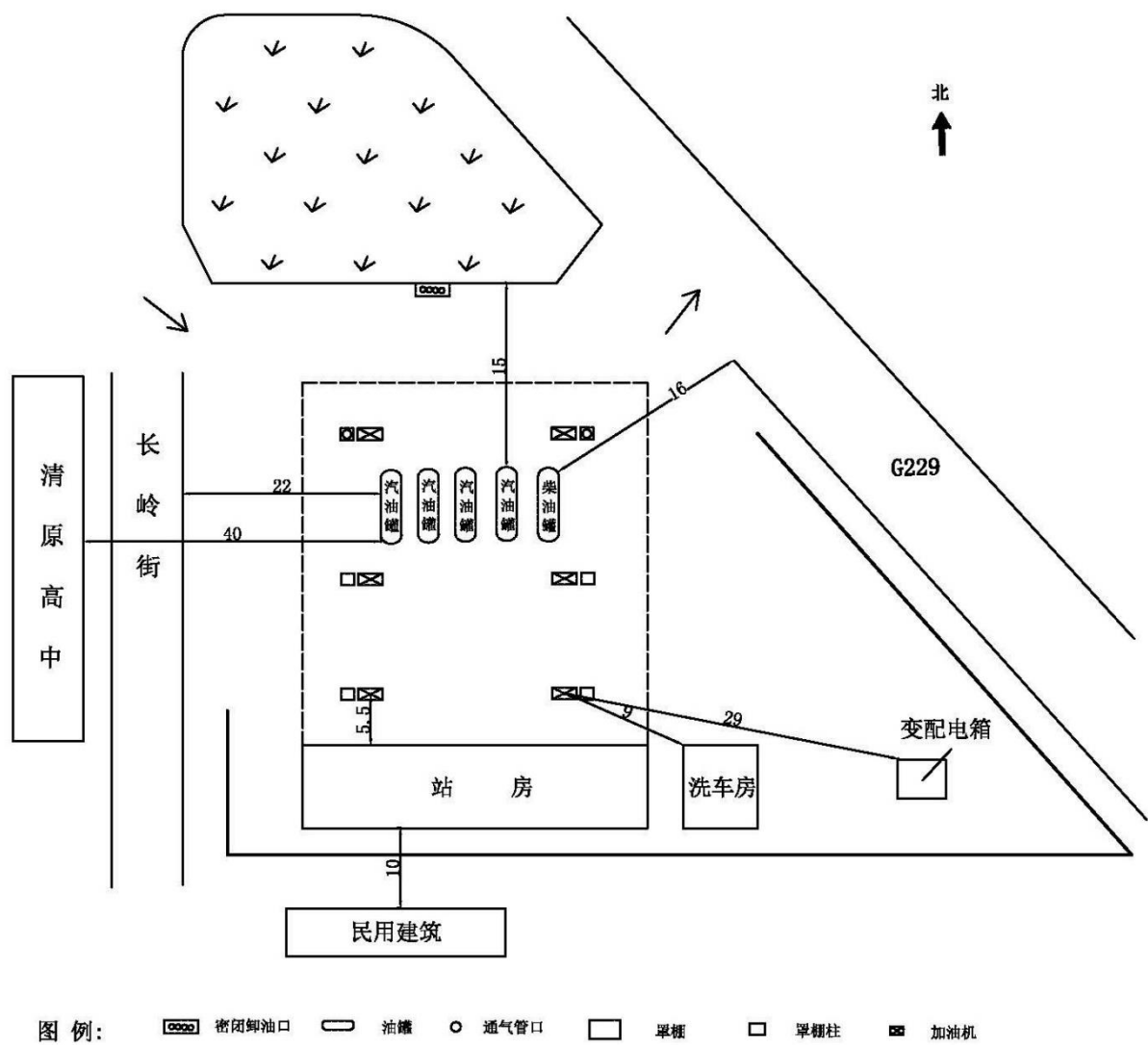
图 2.3-1 加油站周边环境和总平面布置示意图
