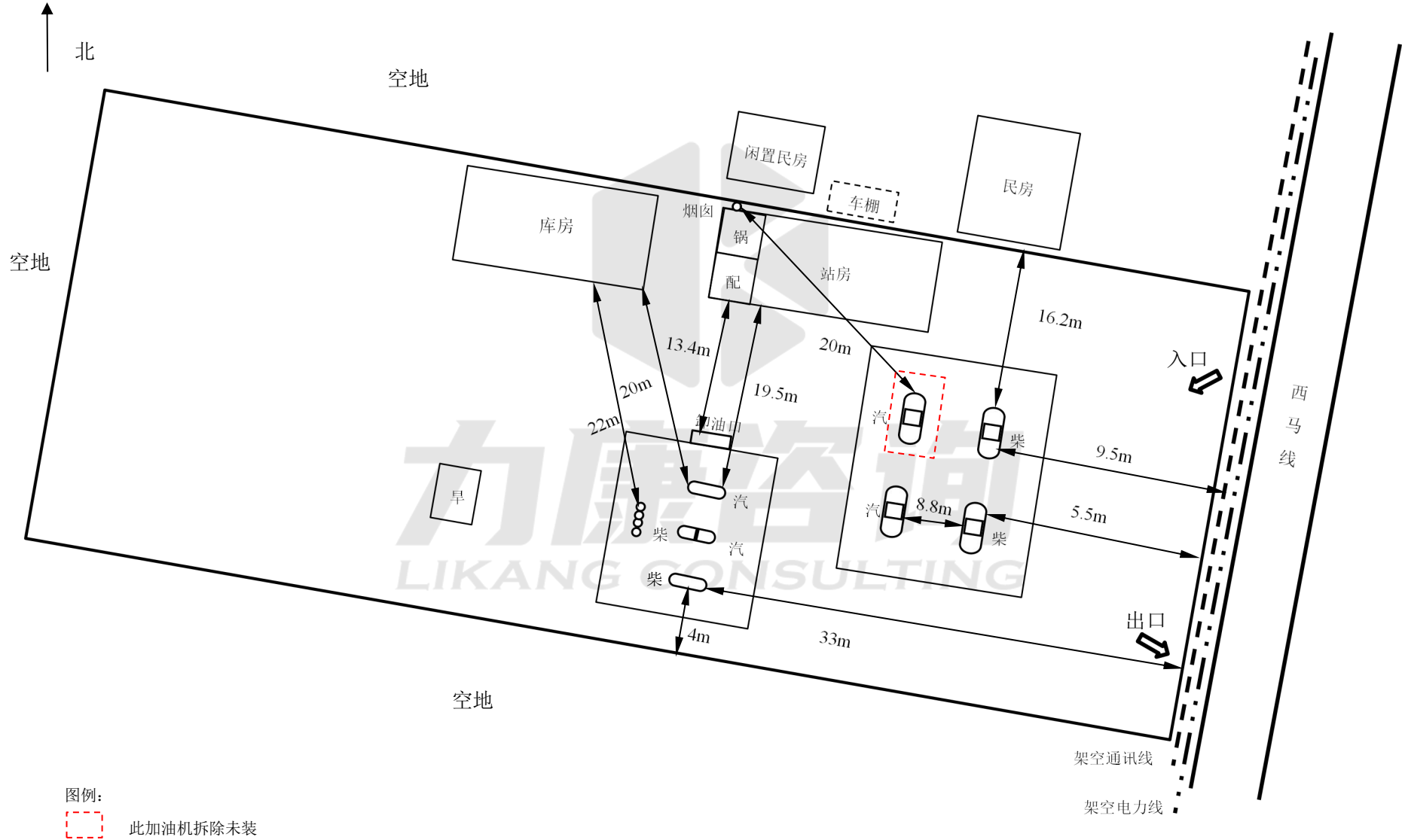
图 2.3-1 周边环境及总平面示意图
